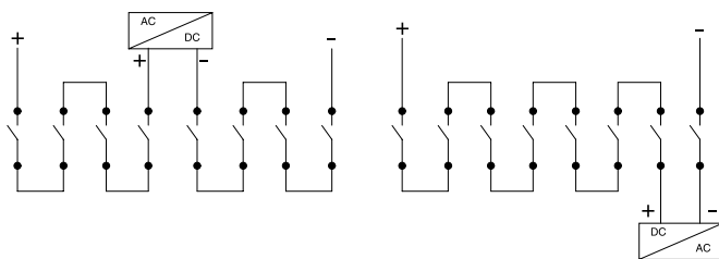
590.DCGE0830 - 590.DCGE0840 - (8 POLI IN SERIE) - 8 PONTICELLI FORNITI
